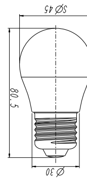
FR34 & FR38 (E27 BASE)
