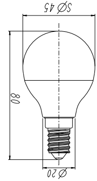
FR36 & FR40 (E14 BASE)
